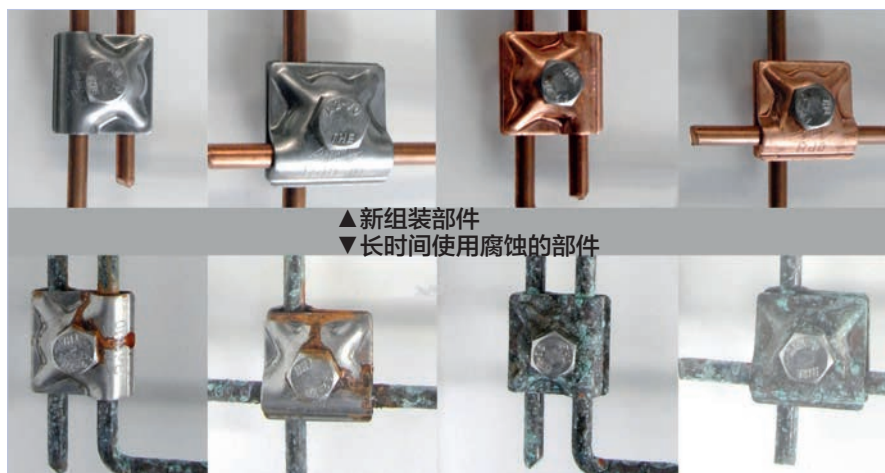
图3: 新部件产品和长时间使用后的对比
