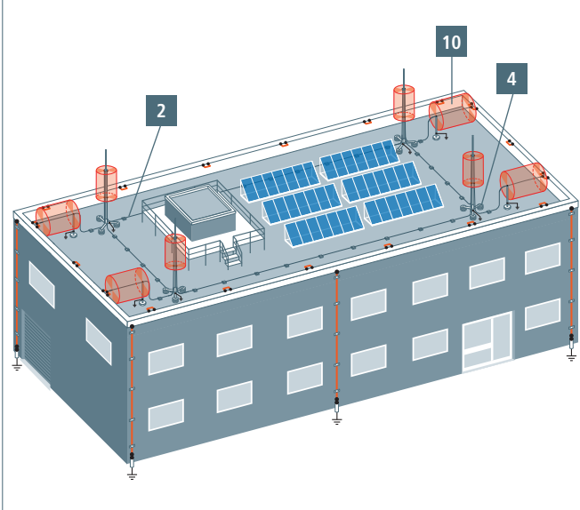
HVI引下线的安装
