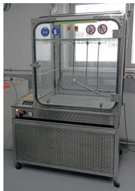
图2: 硫化试验
