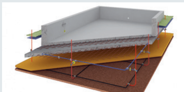
环形接地极
